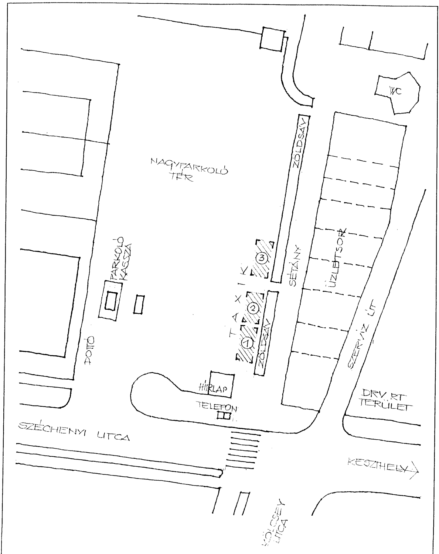
Hévíz , Nagyparkoló tér, helyszínrajz m.1:500 3 db taxi kiállási hely létesítéséhez
