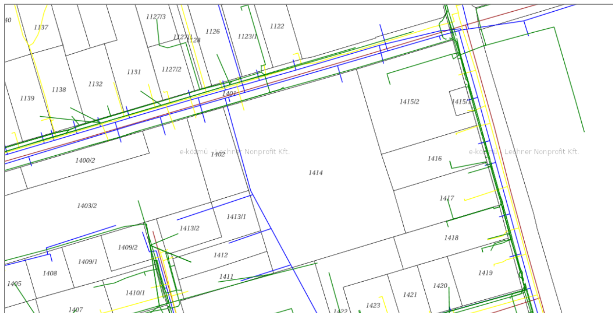
A módosítási terület közműterkép részlete (piros villamos energia, kék vízellátás, sárga szénhidrogén, zöld távközlés, bordó vízvezetés)
