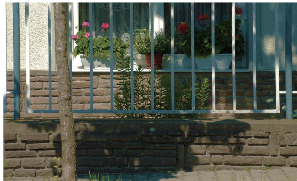
Kerítés kialakítása tömör lábazattal és áttört kerítésmezővel
